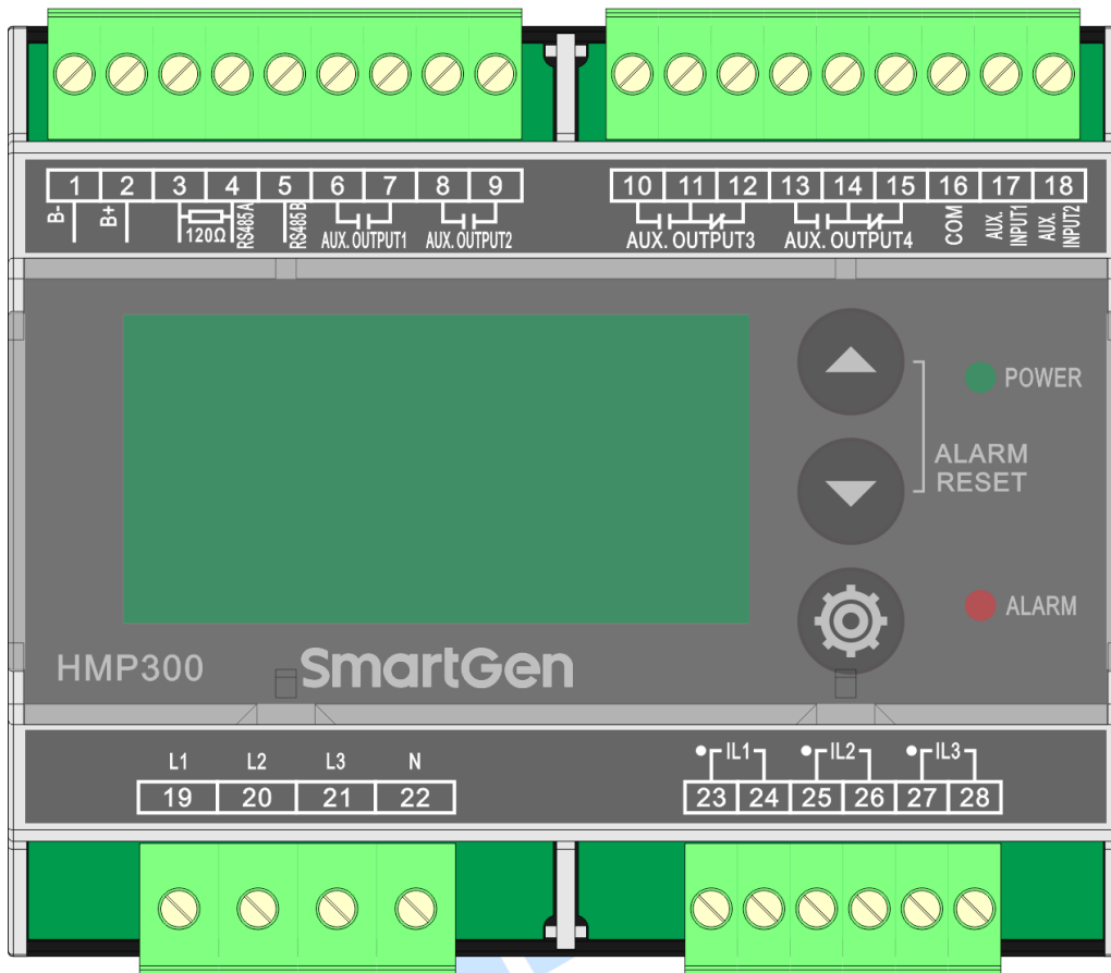
图1 模块面板图
