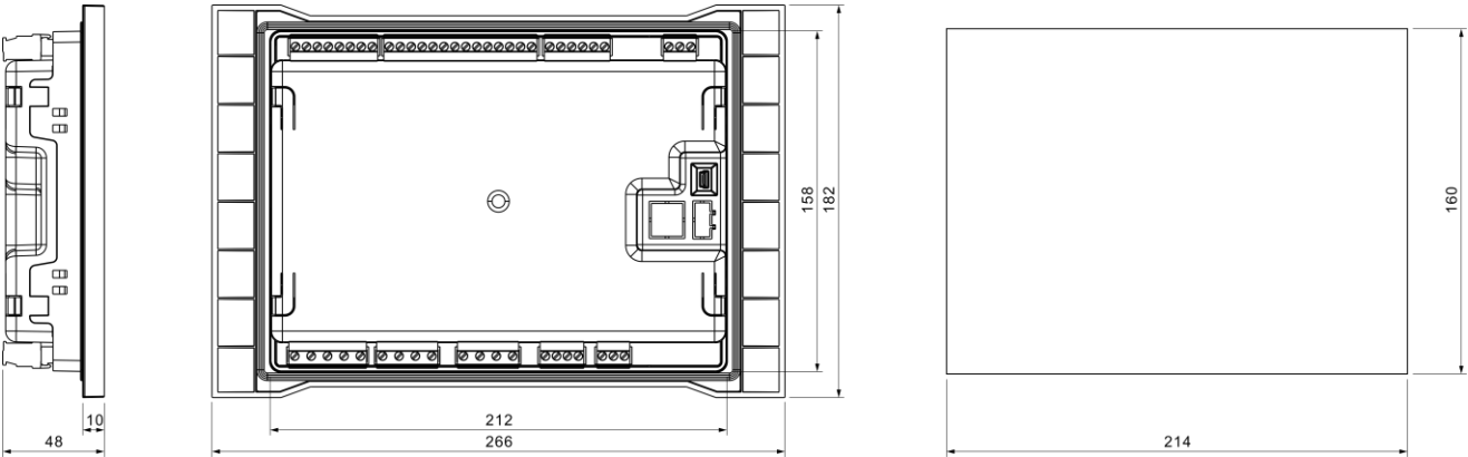
图 11 外形及开孔尺寸
