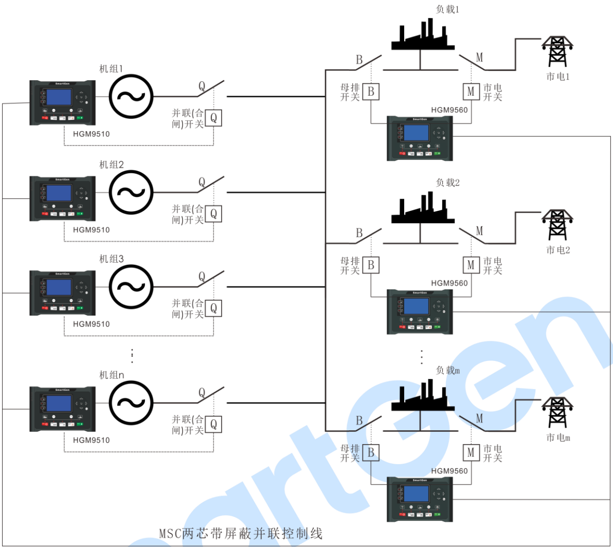
图 10 多路负载应用图
