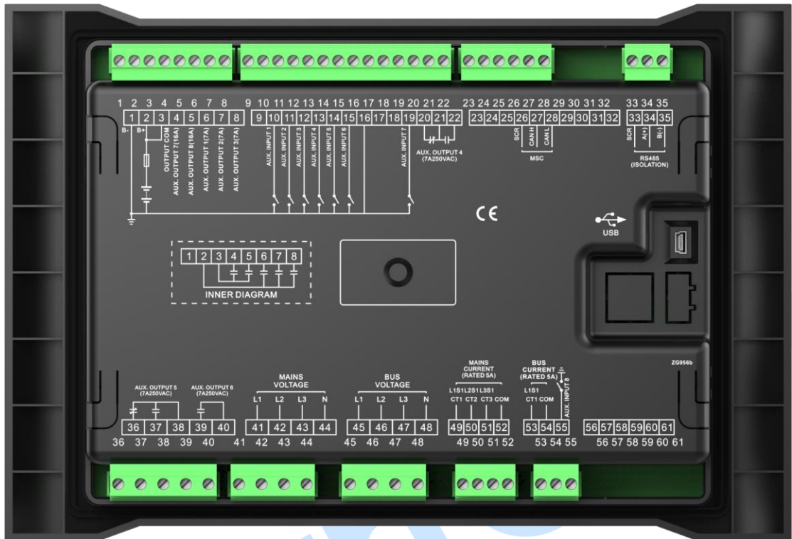
图 2 控制器背面板
