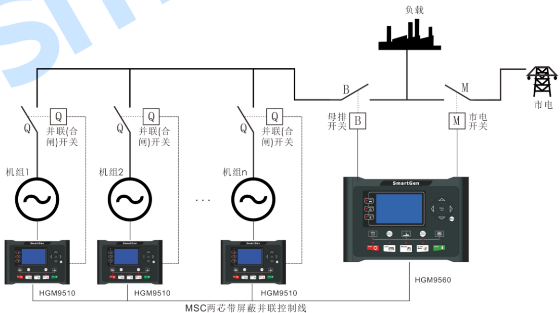
图 9 一路负载应用图
