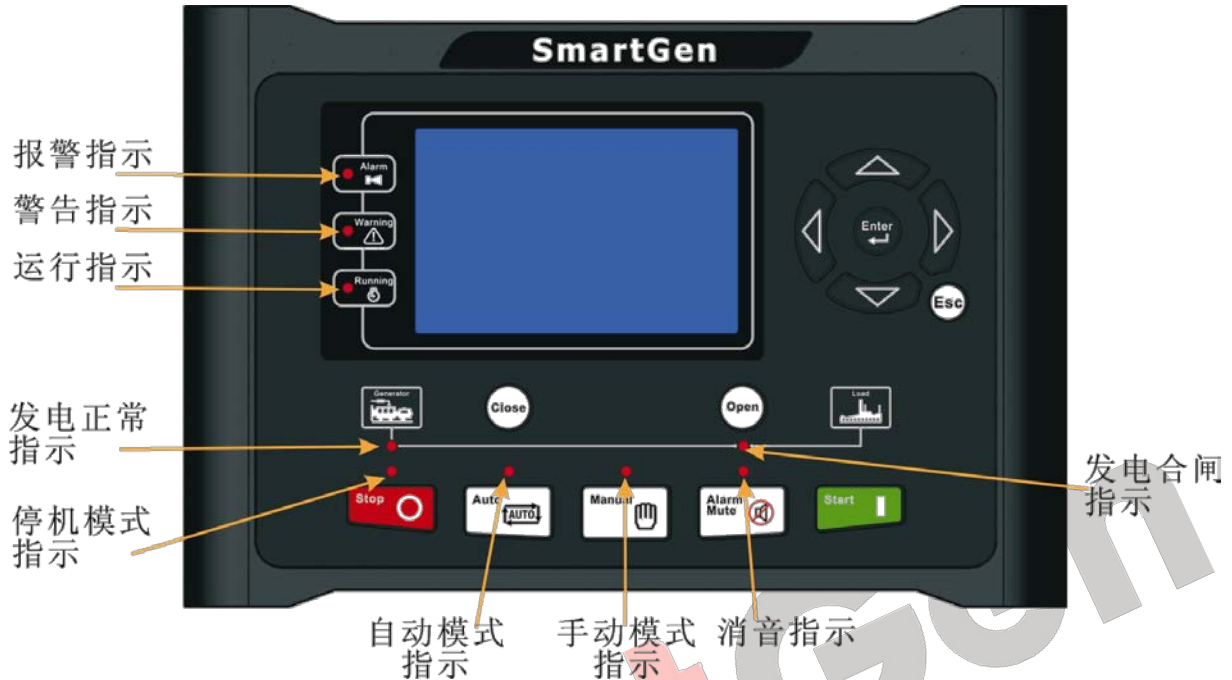
图1 HGM9530 面膜图
