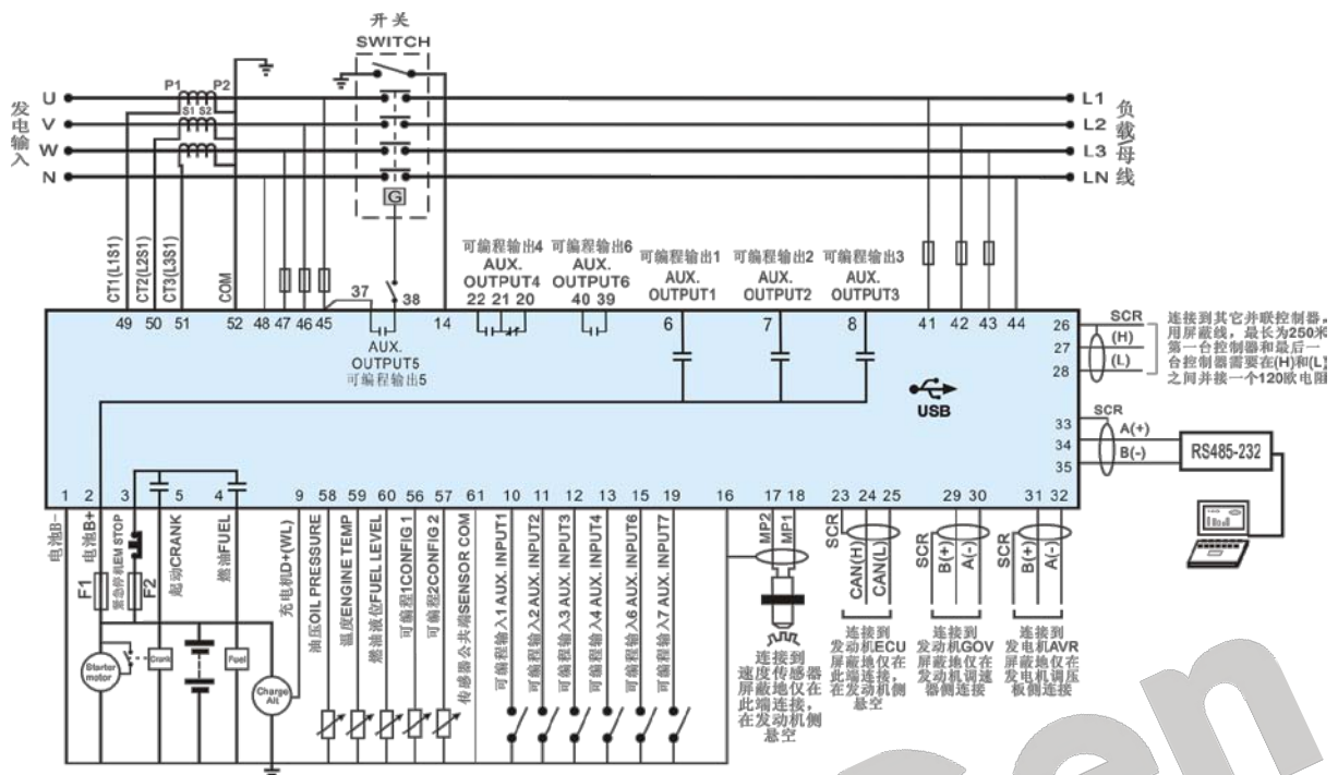
图4 HGM9530 三相四线典型应用图
