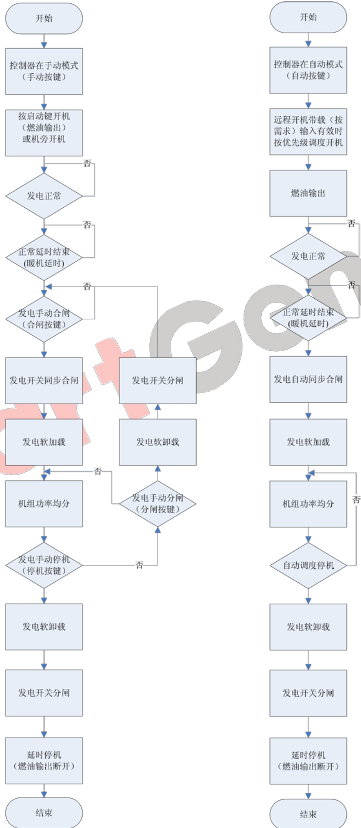
图14 功率管理模式
