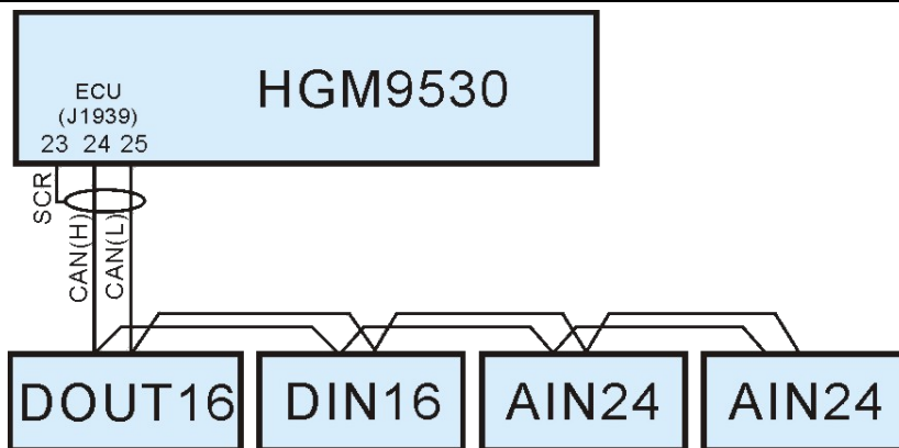
图10 HGM9530 扩展模块连接示意图
