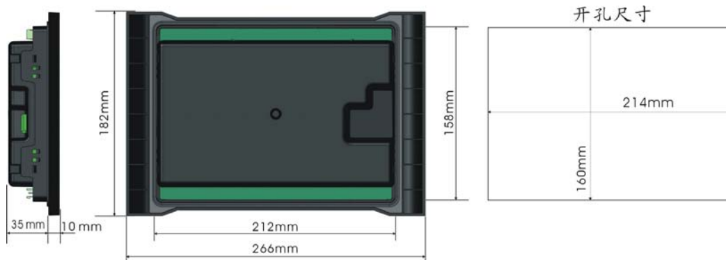
图16 外形尺寸及面板开孔尺寸
