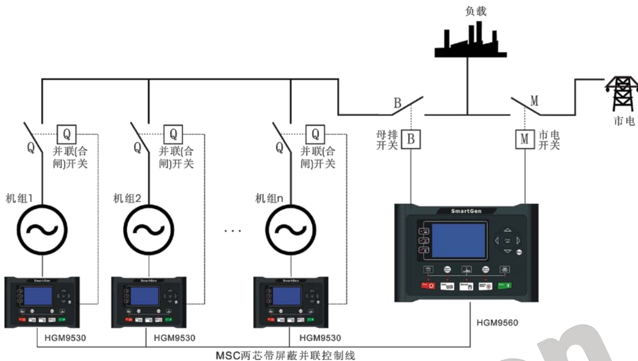
图8 HGM9530 多机并联应用图
