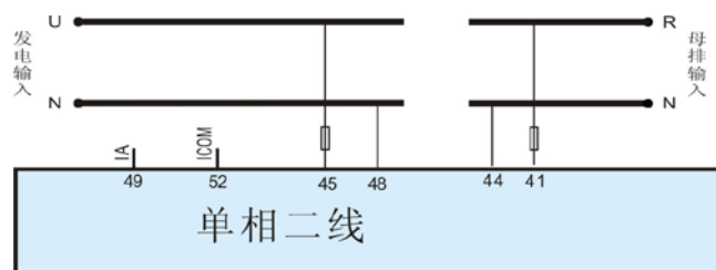
图7 单相二线应用图
