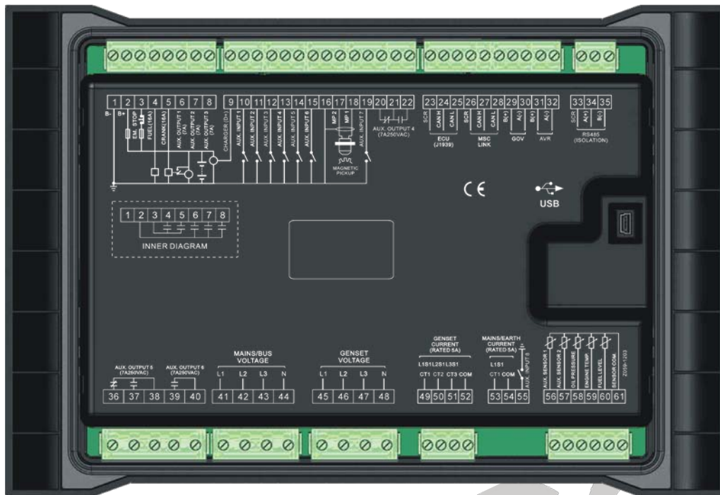
图2 HGM9530 控制器背面板
