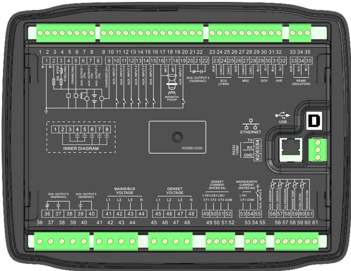
图1 控制器背面板图
