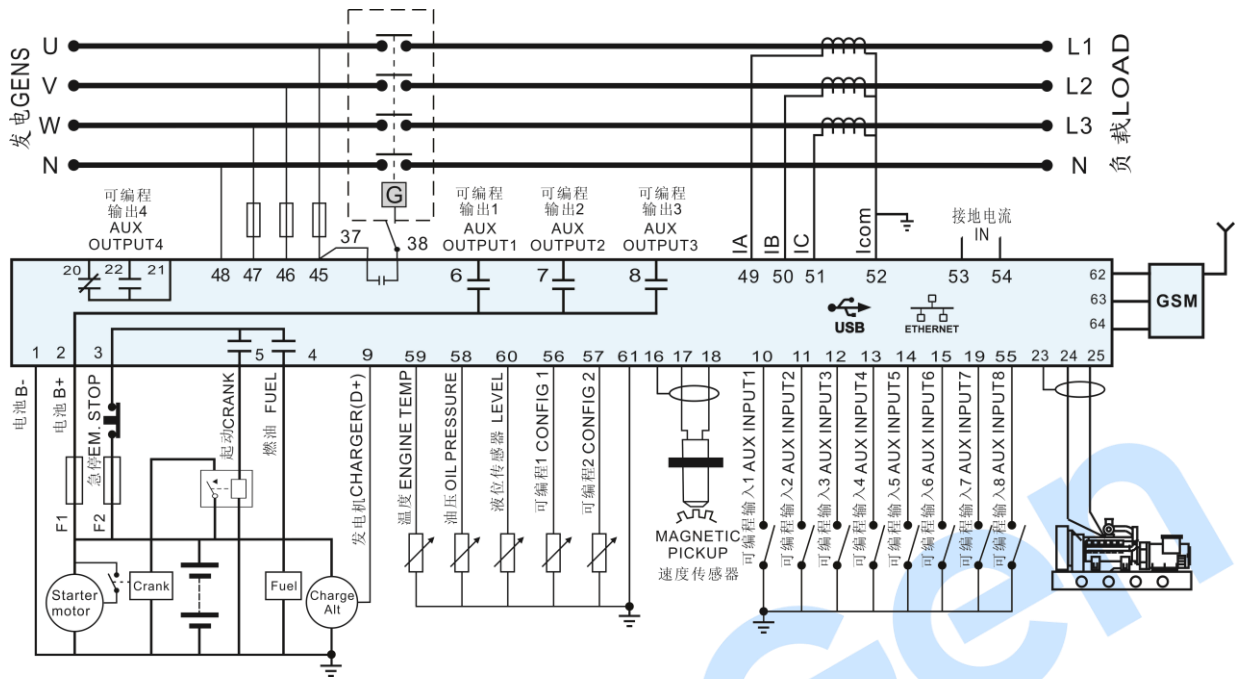
图3 HGM8110N 典型应用图
