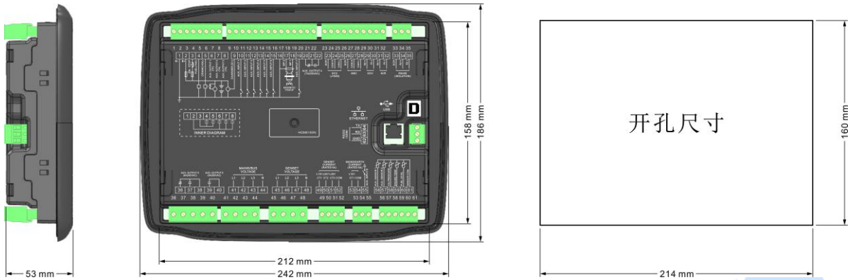
图6 外形及开孔尺寸
