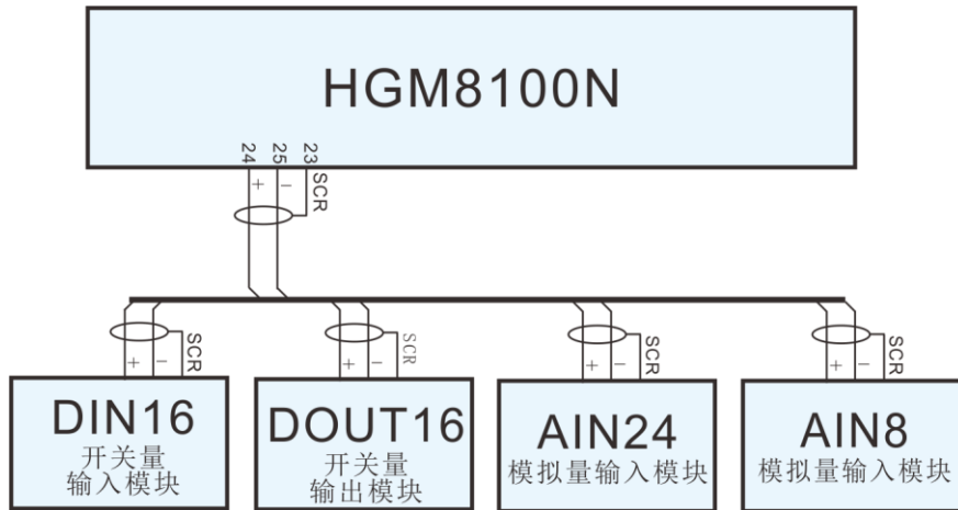
图5 HGM8100N 扩展模块典型应用图
