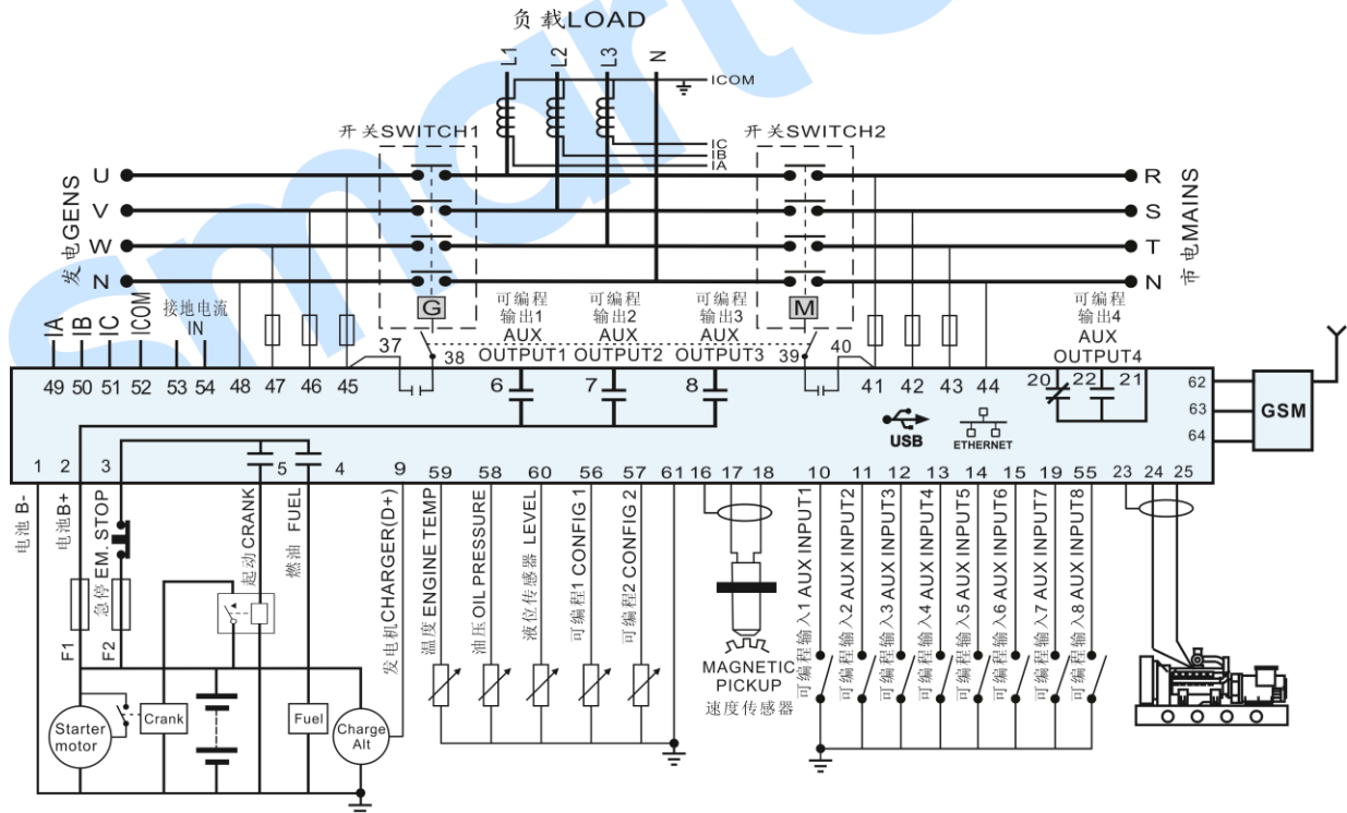
图4 HGM8120N 典型应用图
