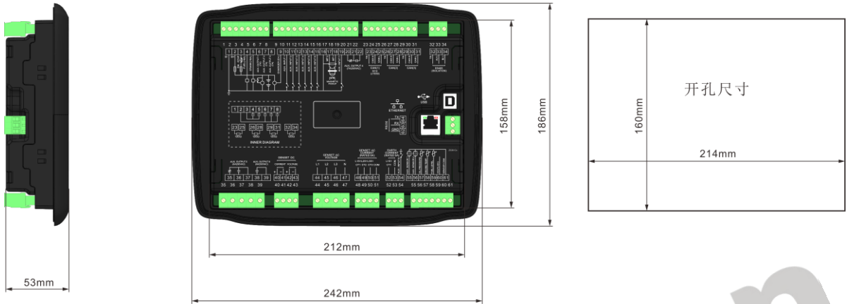
图6 外形及开孔尺寸
