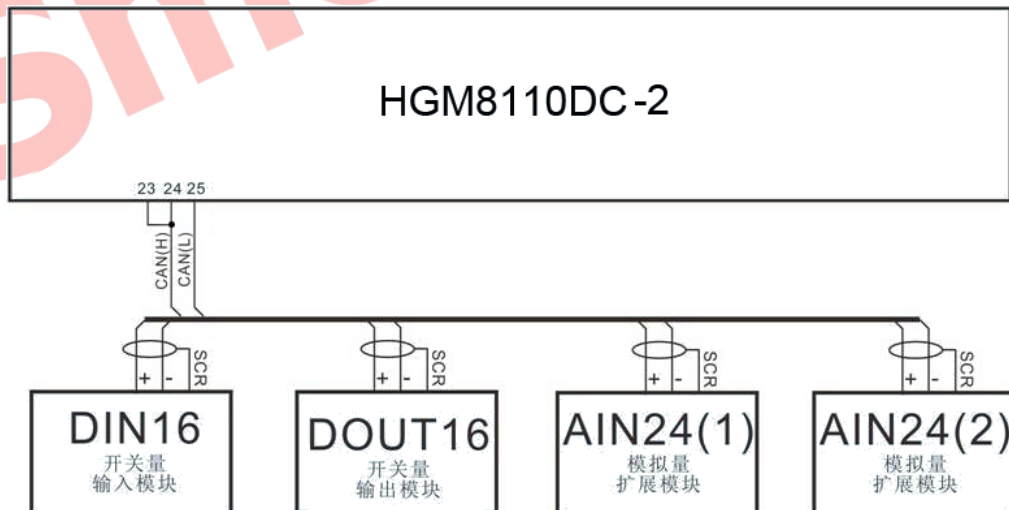
图5 HGM8110DC-2 扩展模块典型应用图
