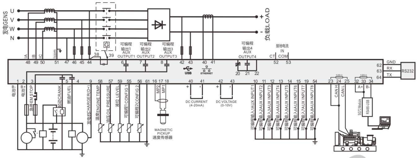
图4 HGM8110DC-2 典型应用图
