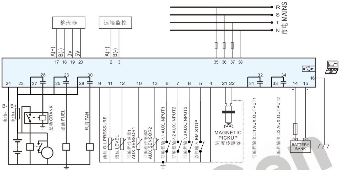
图3 典型应用图
