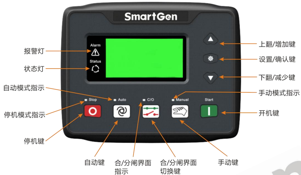
图1 HGM4020DC 前面板指示
