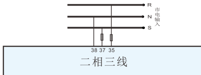
图5 二相三线接线图
