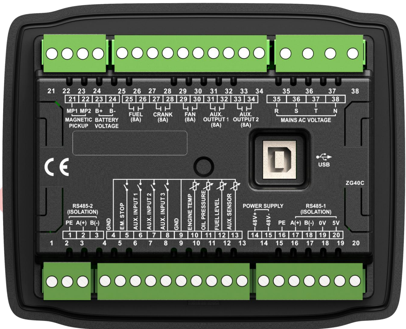
图2 背面板图
