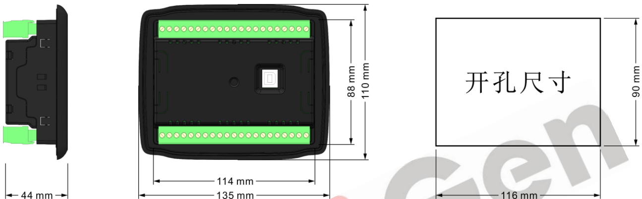
图6 外形及开孔尺寸
