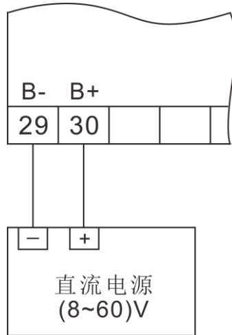
图11 直流供电示意图
