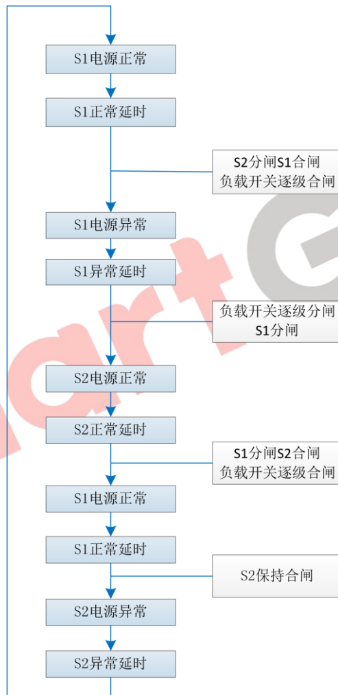
图3 自投不自复流程图
