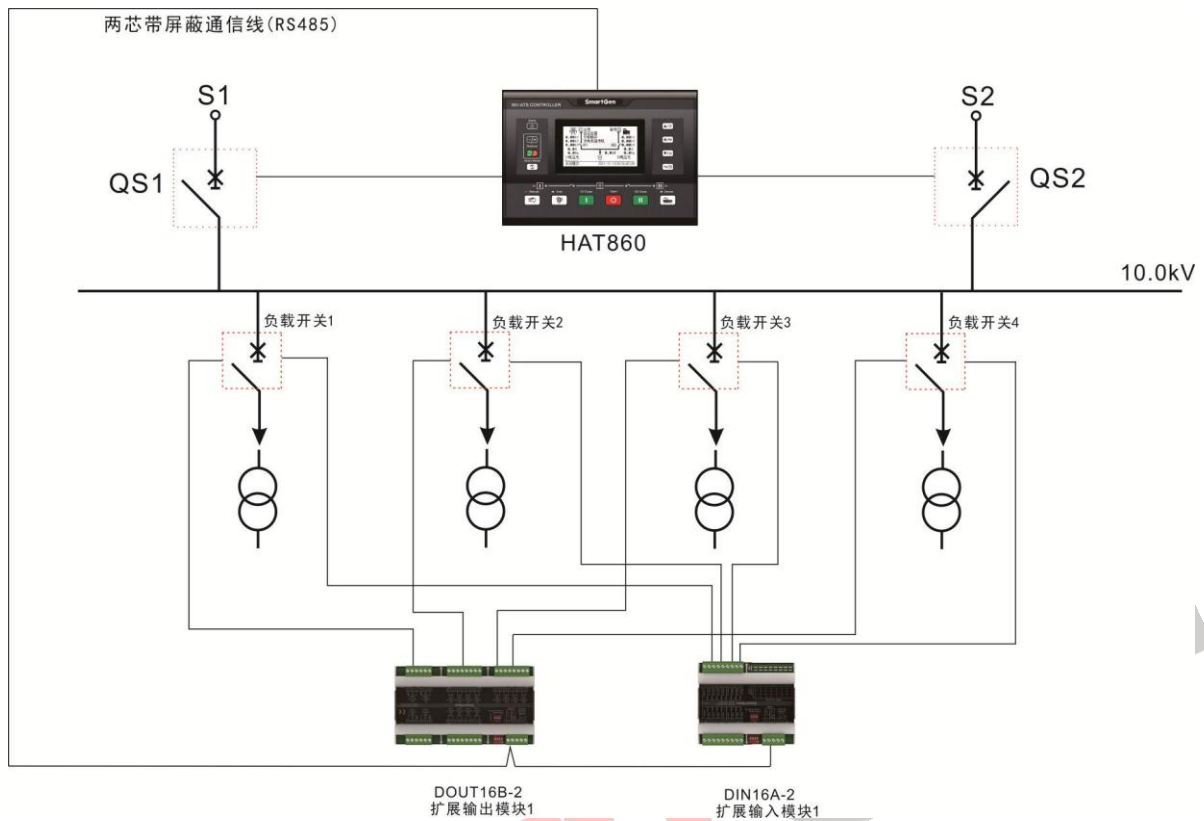
图14 中压负载开关逐级投切控制系统应用图
