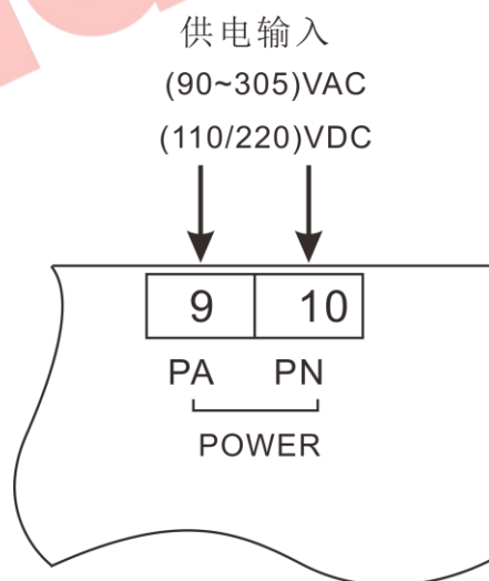
图10 供电示意图
