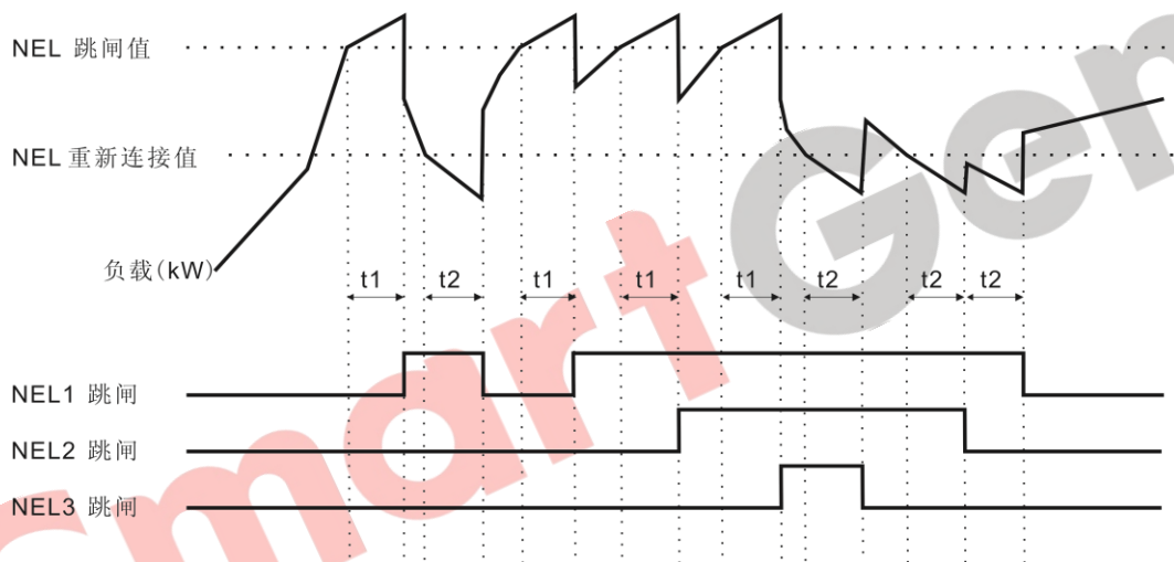
图5 NEL 跳闸
