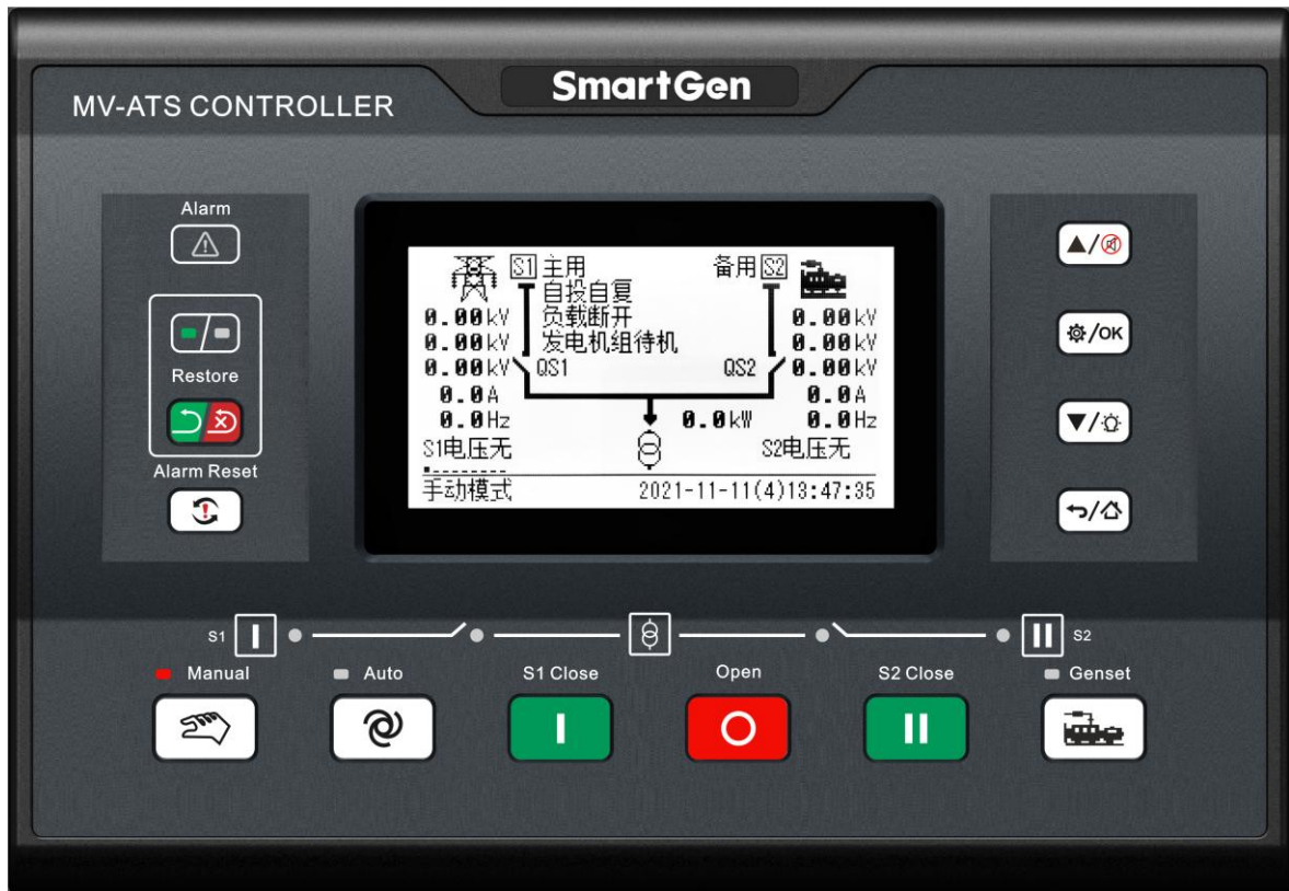
图1 面板指示图
