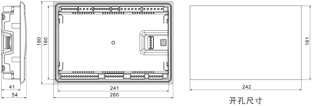
图16 外形尺寸及面板开孔尺寸
