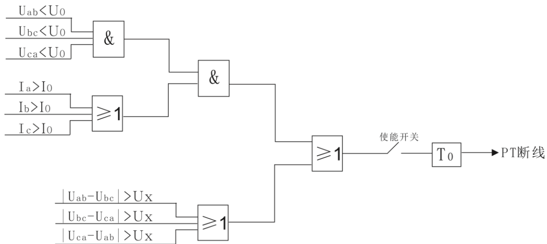
图4 PT 断线检测逻辑图
