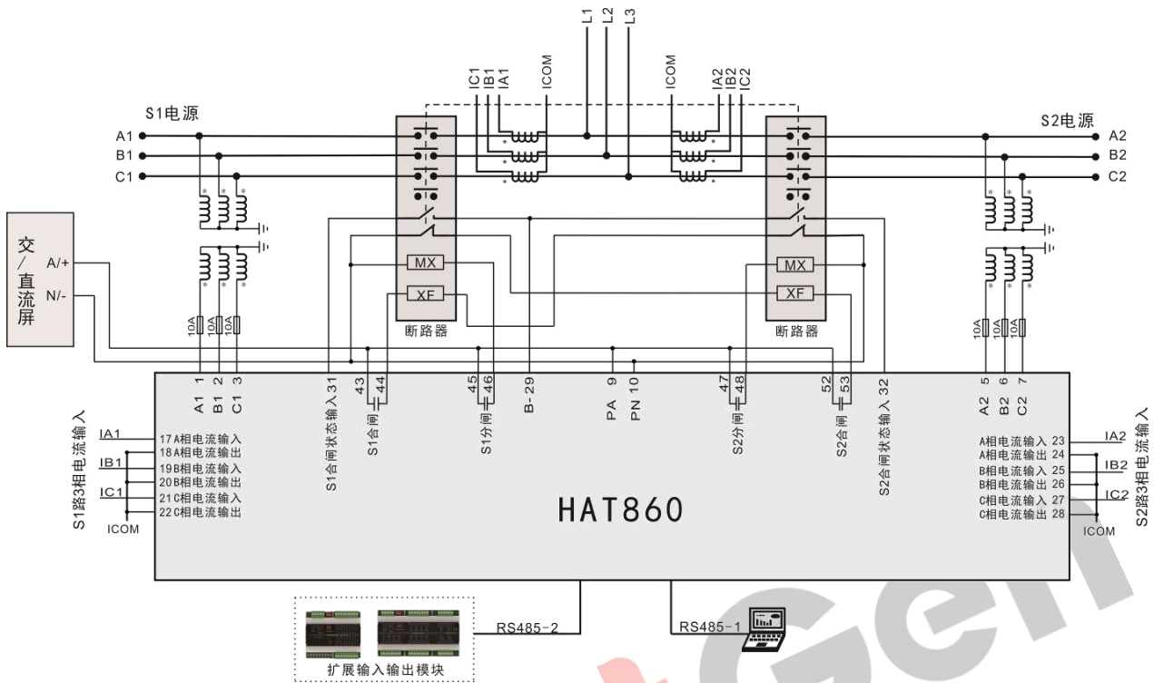
图13 断路器应用图
