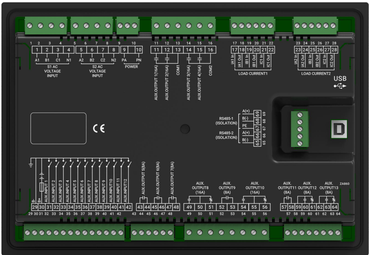
图9 控制器后面板图
