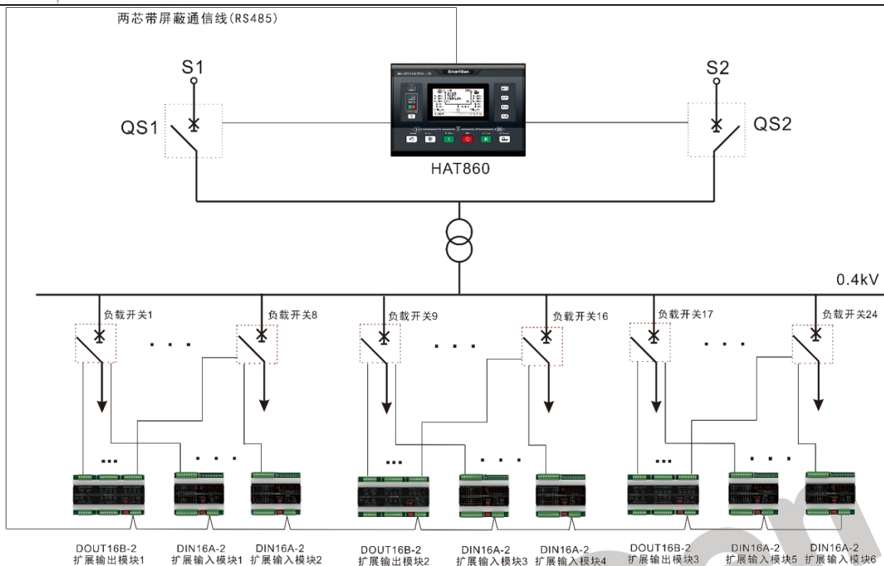
图15 低压负载开关逐级投切控制系统应用图
