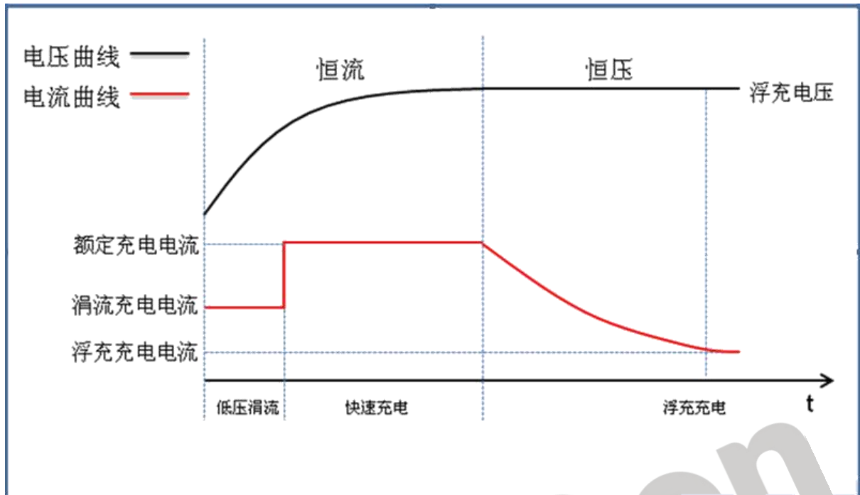
图2 二段式充电曲线图
