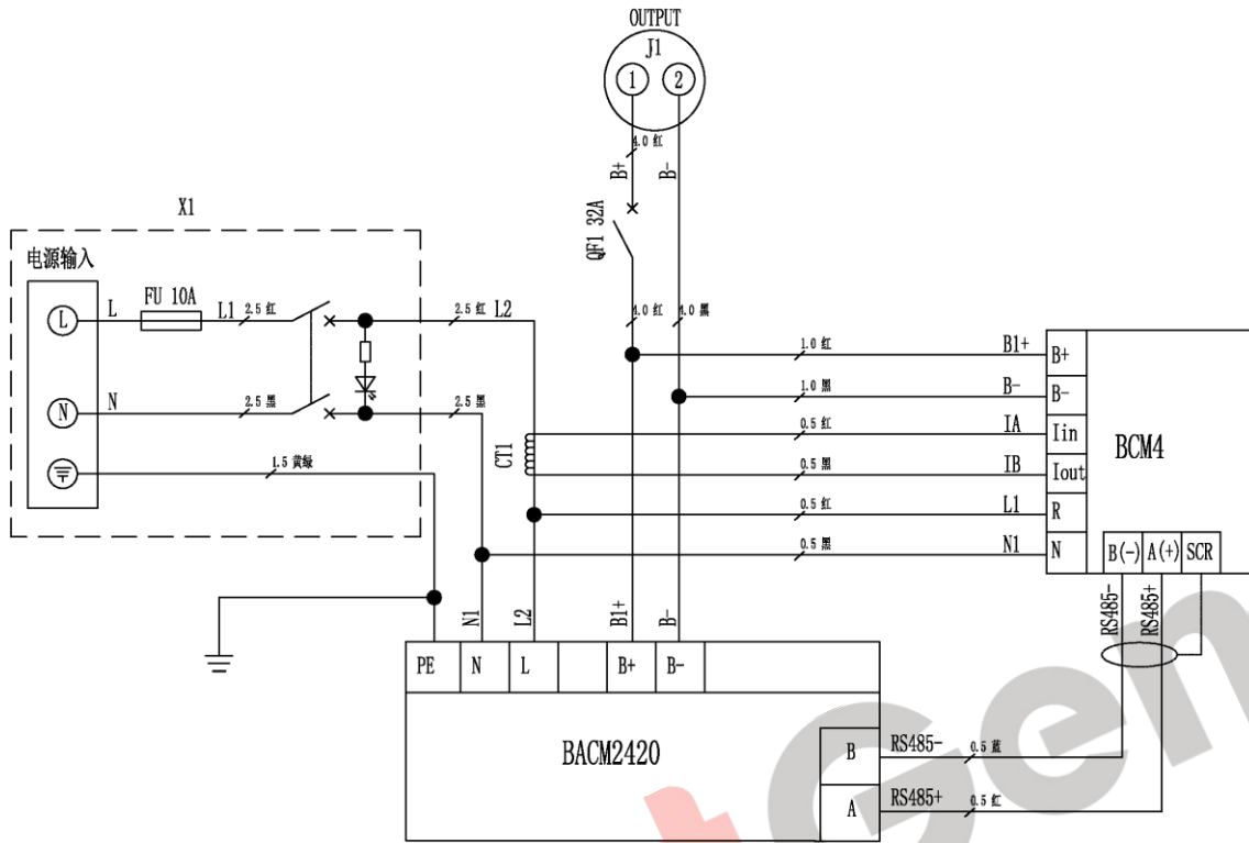
图5 充电器和控制器内部接线图
