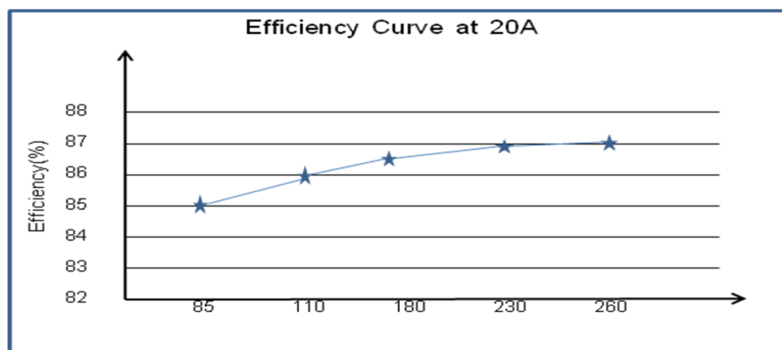
图3 效率曲线
