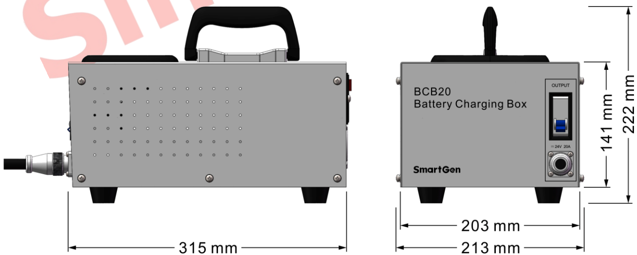
图6 外形尺寸图
