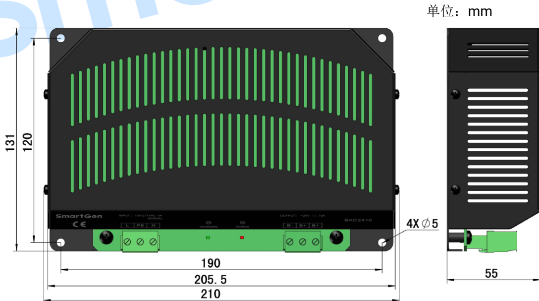
图4 BAC2410 安装尺寸图
