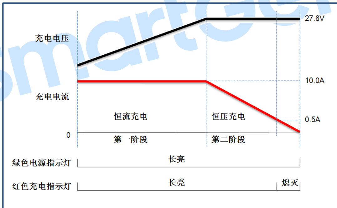
图1 二阶段式充电曲线图
