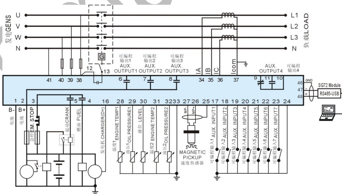
HGM6210KC 典型应用图
