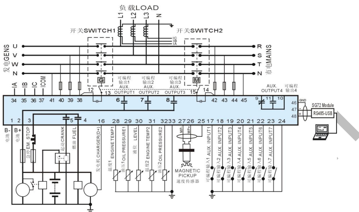
单相二线连接时接线图(以 HGM6220KC 为例)
