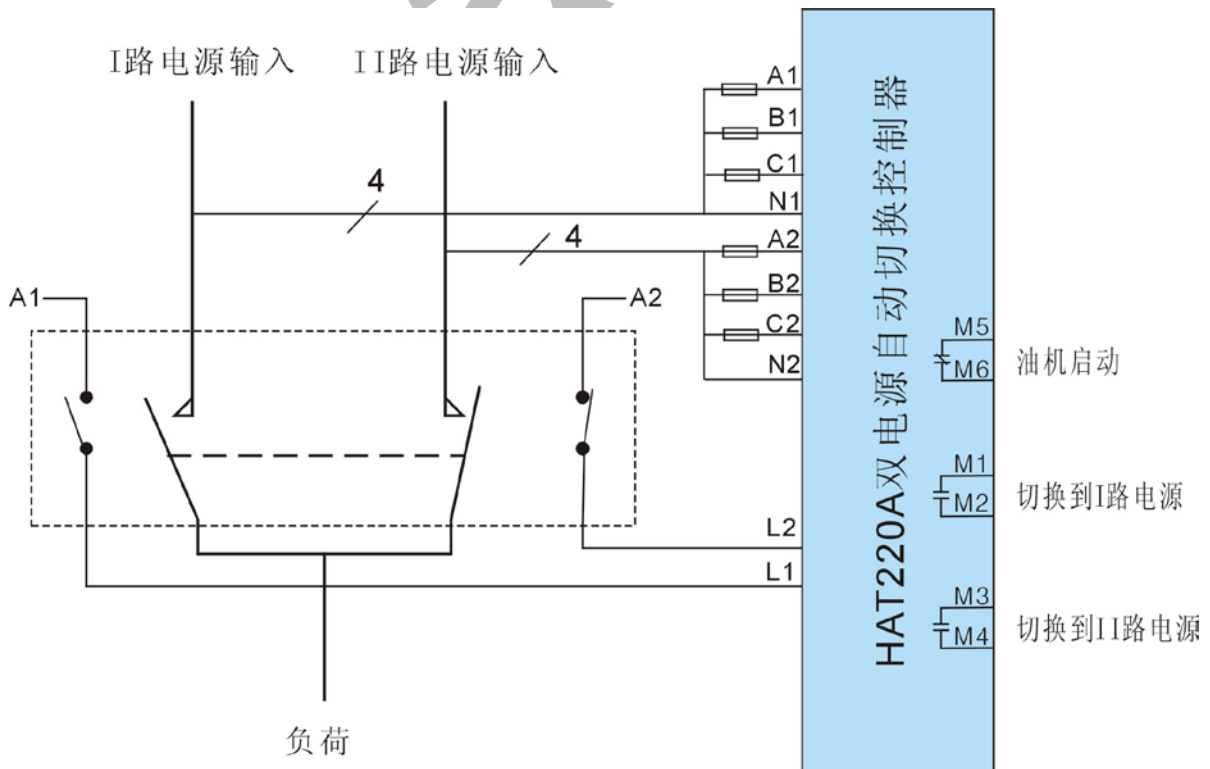
HAT220A 应用接线图
