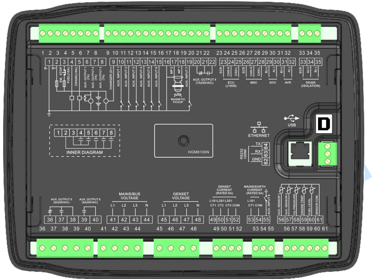
图1 控制器背面板图
