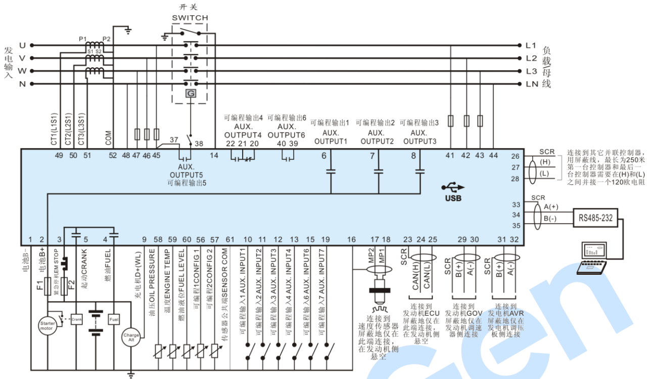
图3 HGM8151 三相四线典型应用图
