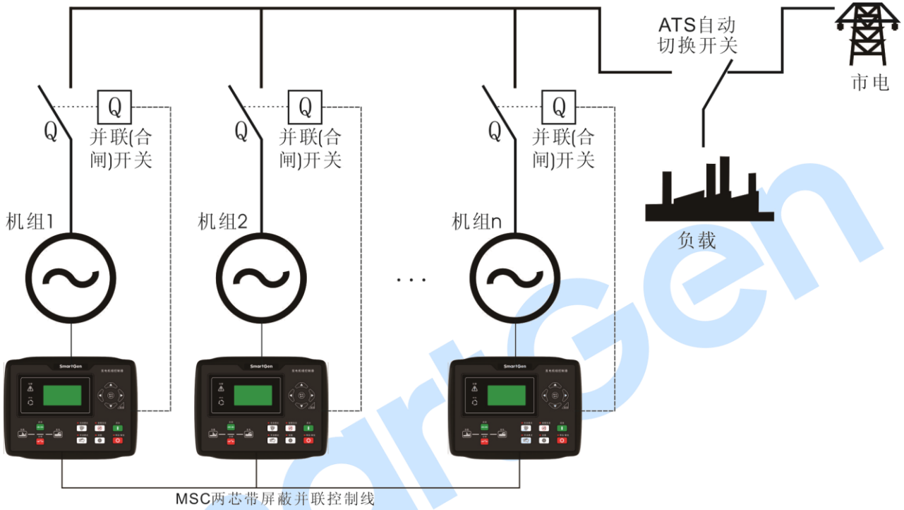
图7 HGM8151 多机并联应用图
