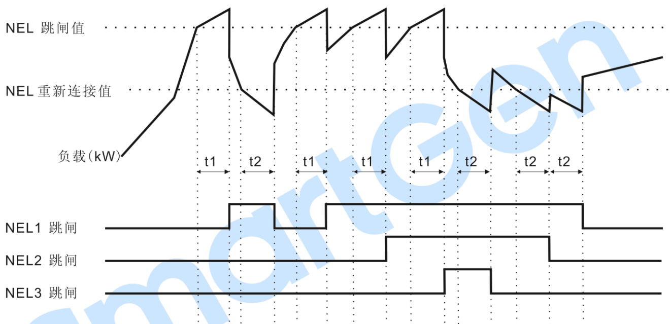
图10 非重要负载跳闸示意图
