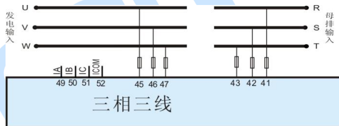
图4 HGM8151 三相三线典型应用图
