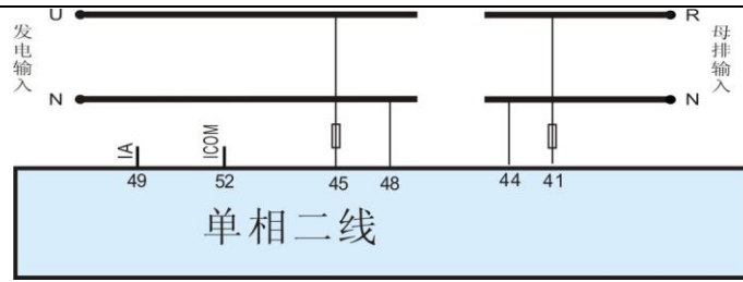
图6 HGM8151 单相二线典型应用图
