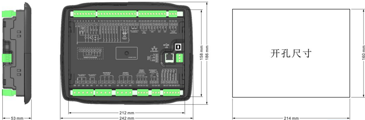
图11 外形及开孔尺寸
