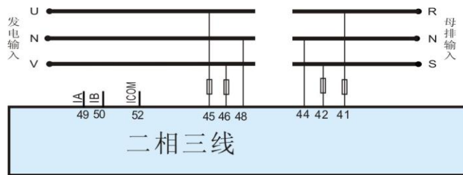
图5 HGM8151 二相三线典型应用图
