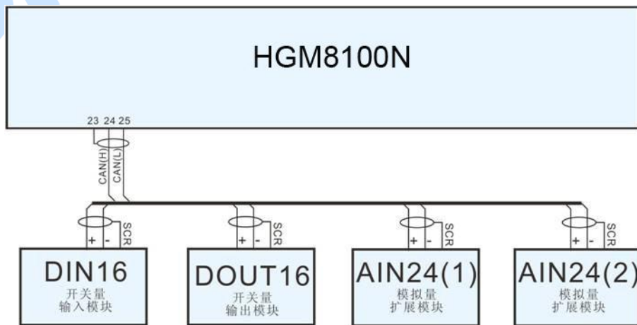
图8 HGM8151 扩展模块典型应用图
