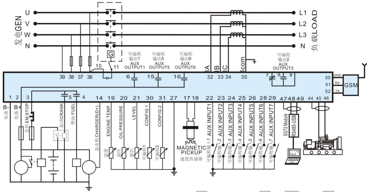
HGM7210CAN 典型应用图
