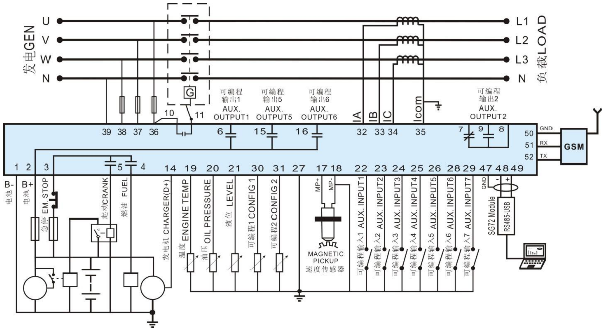
HGM7210 典型应用图
