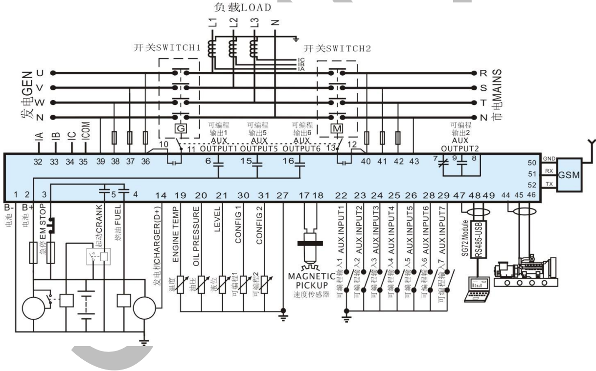
HGM7220CAN 典型应用图
