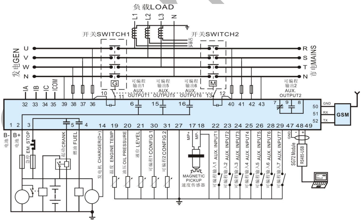
HGM7220 典型应用图
