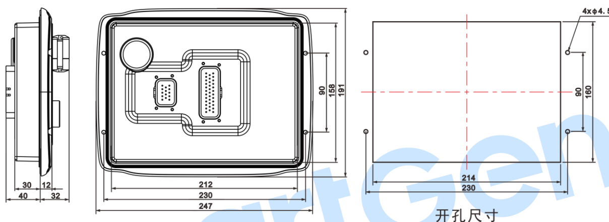
图7 外形及开孔尺寸
