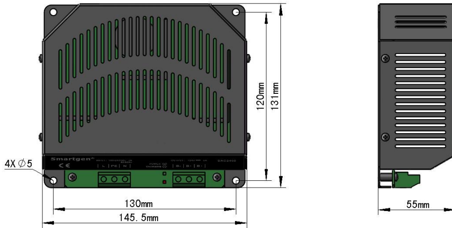
图 4 BAC2408 安装尺寸图
