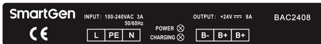
图 3 BAC2408 面板图
