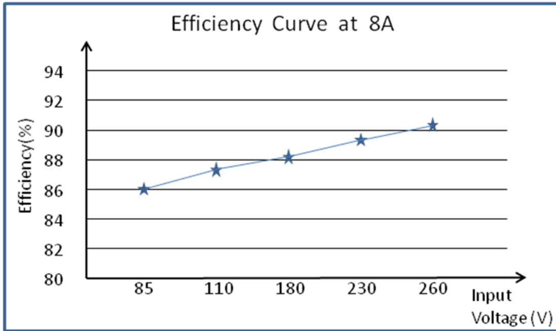
图 2 效率曲线
