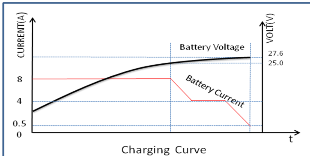
图 1 充电原理图
