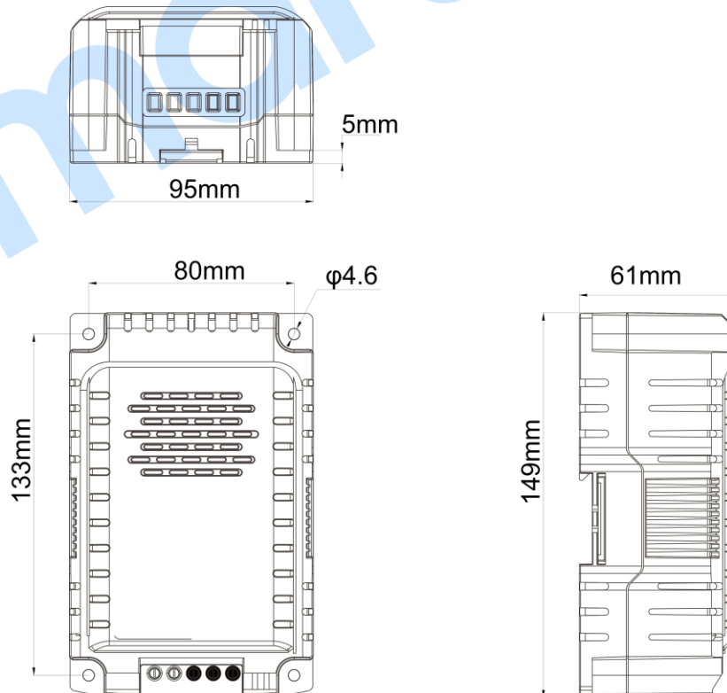
图3 螺丝固定安装
