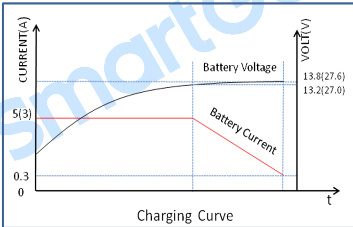
图1 充电原理图
