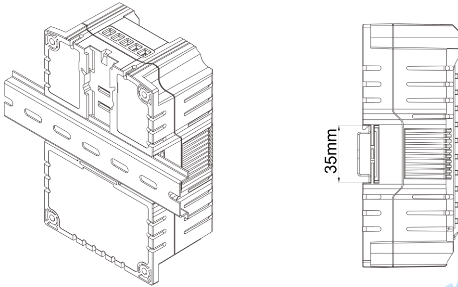
图4 导轨安装
