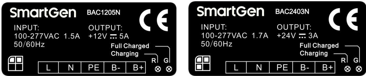
图2 BAC1205N（左）和 BAC2403N（右）面板图
