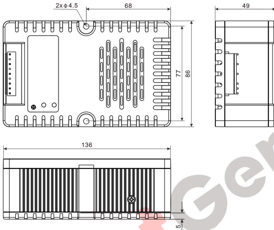
图6 安装尺寸图
