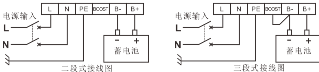
图5 BAC06PB 接线图
