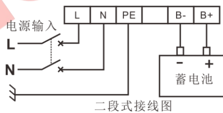
图4 BAC06P 接线图
