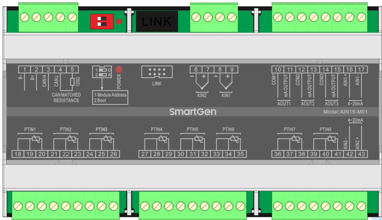
图1 AIN16-M01 端子图
