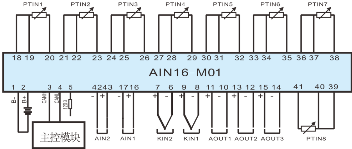
图2 电气接线图
