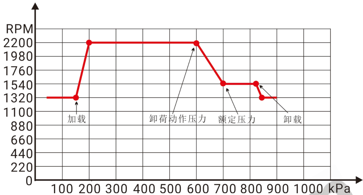
图2 转速-压力曲线图
