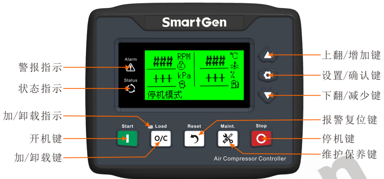
图1 前面板图
