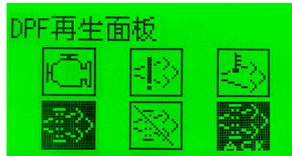
图4 DPF 再生准备就绪
